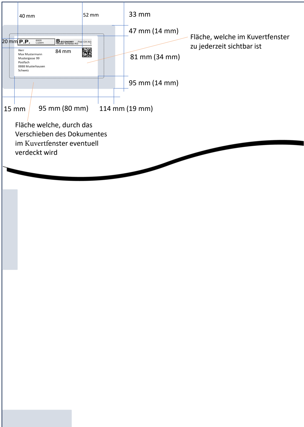
Ansicht der Fenster-Position und der PP-Zeile mit dem Standard-Fenster Kuvert C5 Fenster Links (Fenstergrösse 50 x 100 mm) mit einem A4, Messpunkt obere Kante Links
